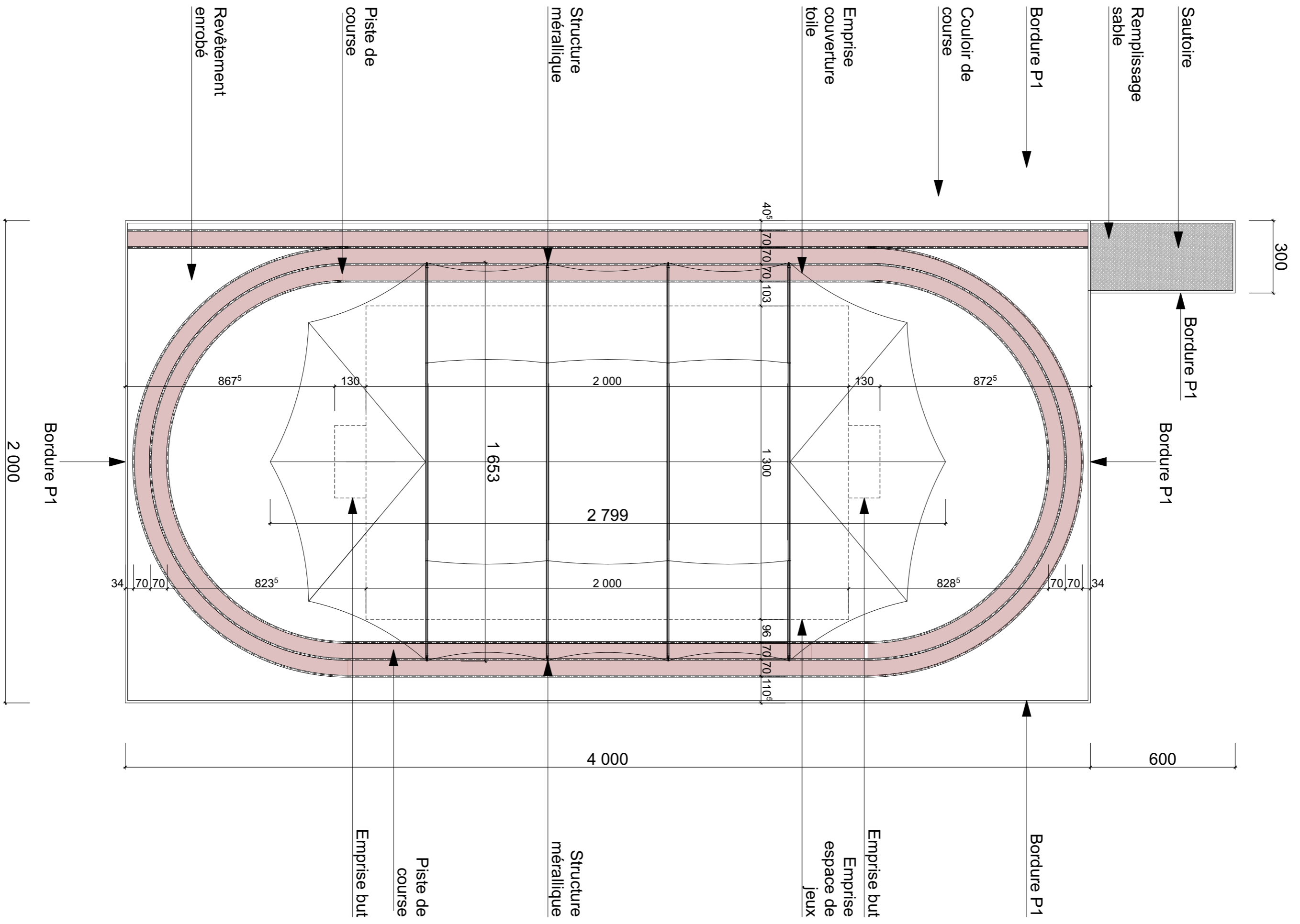
Plan masse de la piste 1/150°
